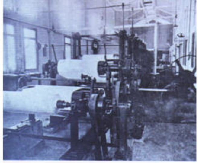
(ซ้าย) โรงงานกระดาษไทย จังหวัดกาญจนบุรี เป็นอีกแห่งที่ใช้ผลิตกระดาษสำหรับพิมพ์ธนบัตร (ขวา) เครื่องจักรทำกระดาษภายในโรงงาน
